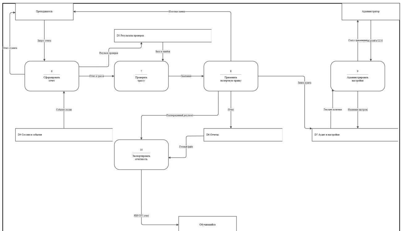
Рис. 32. DFD уровня 2: отчетность и администрирование
