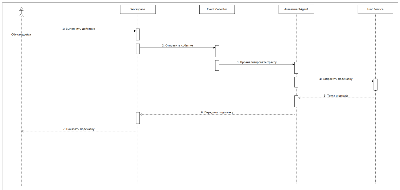
Рис. 13. Диаграмма последовательности обработки инцидента и подсказки Проверка результата и формирование отчета показаны на Рис. 14. Verification Engine запускает checks, AssessmentAgent рассчитывает балл, Reports API формирует отчет.
