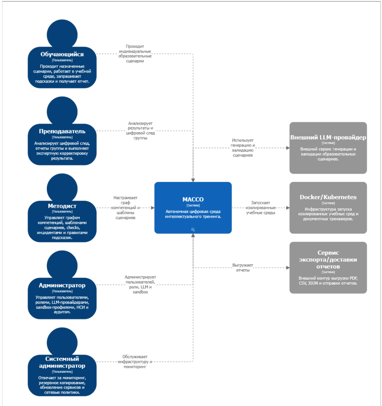
Рис. 25. C4 Context: MACCO во внешней среде
