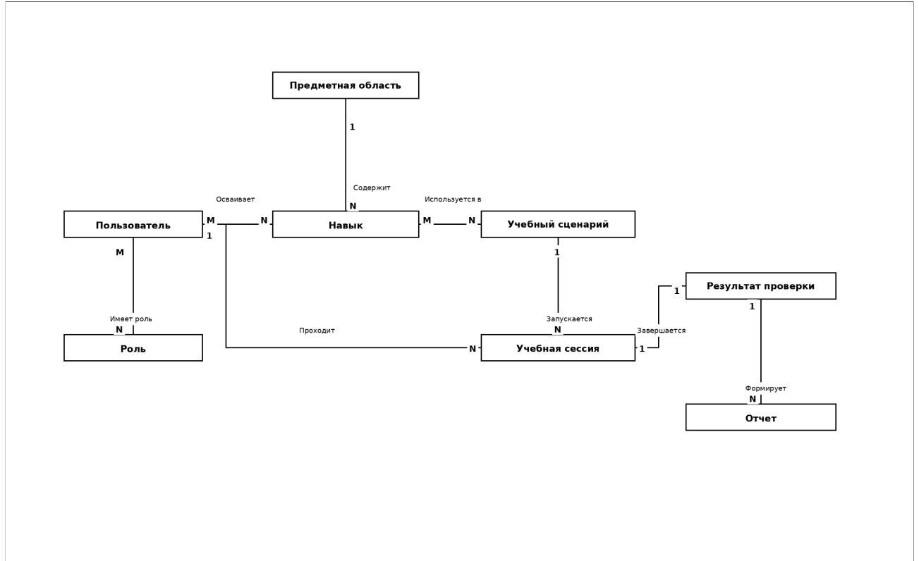
Рис. 19. Концептуальная модель данных
