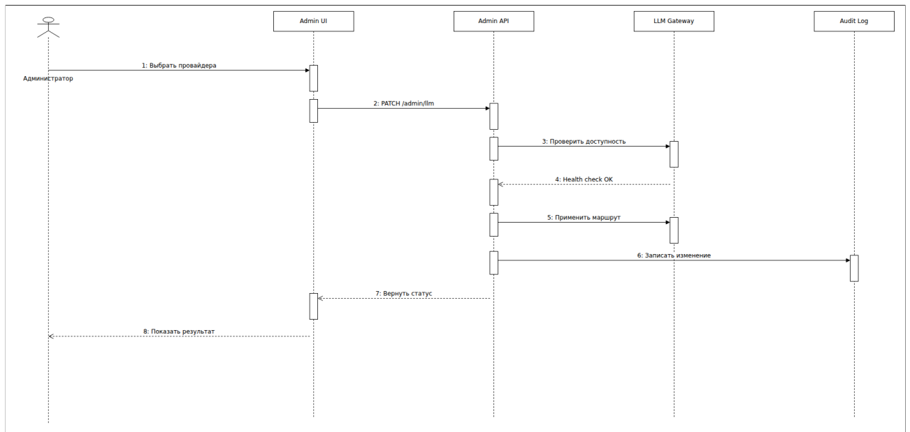
Рис. 17. Диаграмма последовательности переключения LLM-контура
