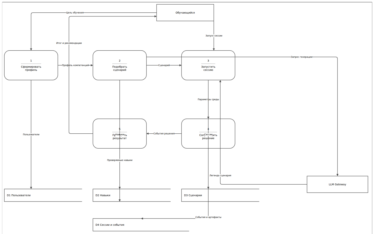
Рис. 31. DFD уровня 1: жизненный цикл обучения
