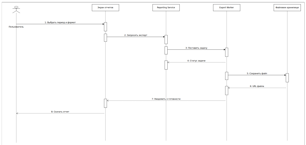
Рис. 18. Диаграмма последовательности экспорта отчетности
