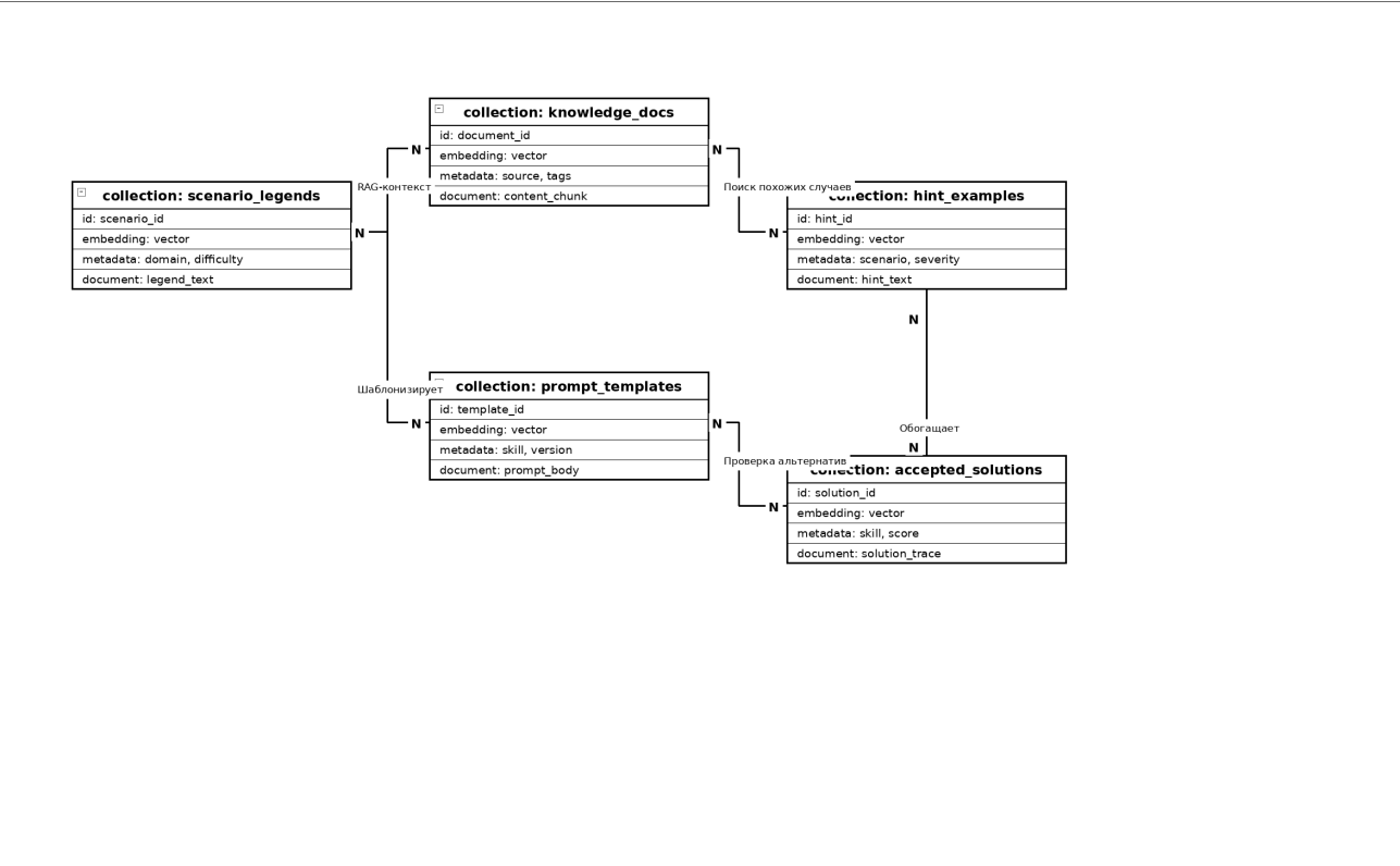
Рис. 23. Физическая модель данных ChromaDB
