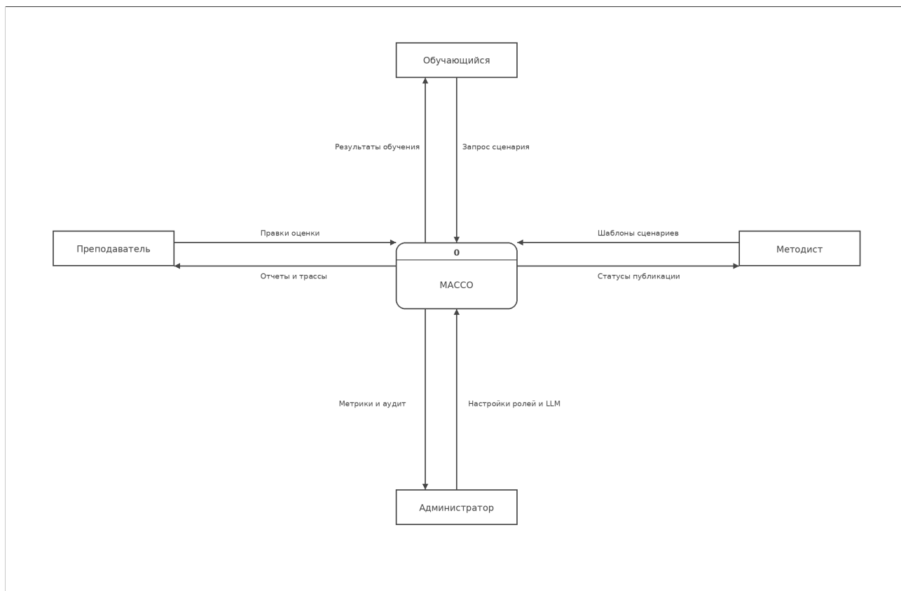
Рис. 30. Контекстная DFD MACCO
