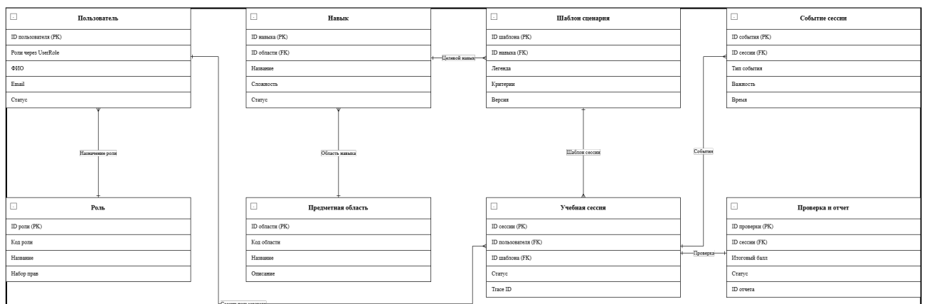
Рис. 20. Логическая модель данных
