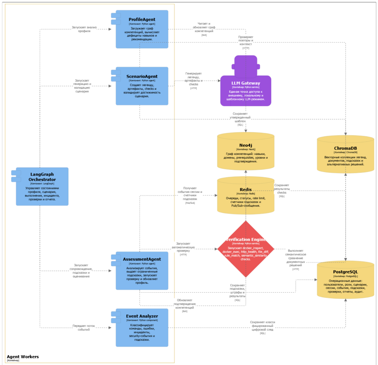
Рис. 28. C4 Component: backend и агенты
