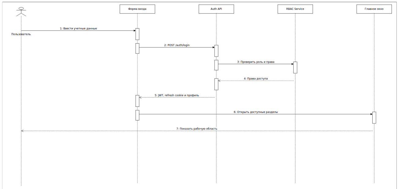
Рис. 9. Диаграмма последовательности входа пользователя
